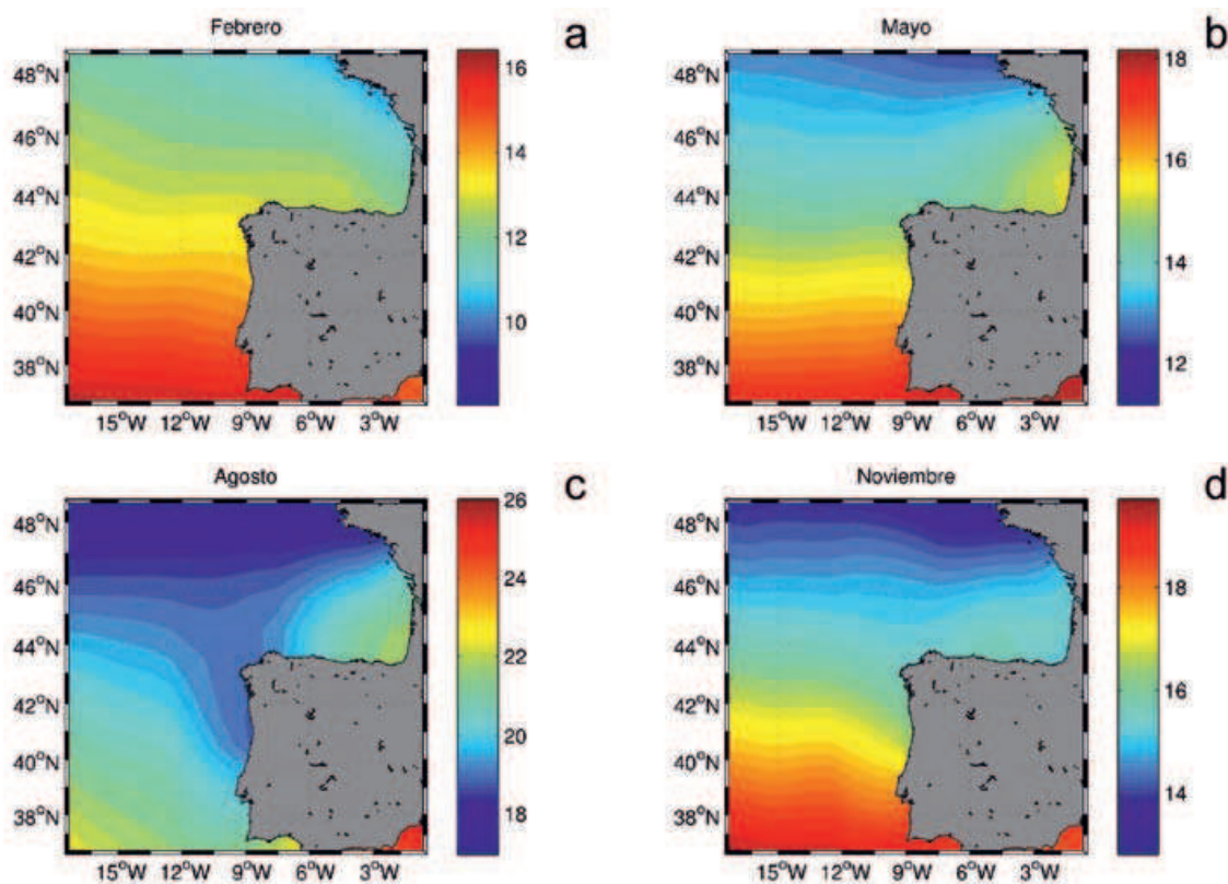
Figura 2.5. Promedio de largo término de la señal SST (°C) en el Golfo de Vizcaya en febrero (a), mayo (b), agosto (c) y noviembre (d), a partir de la base de datos NOAA_OI_SST_V2 entre 1980 y 2009.
