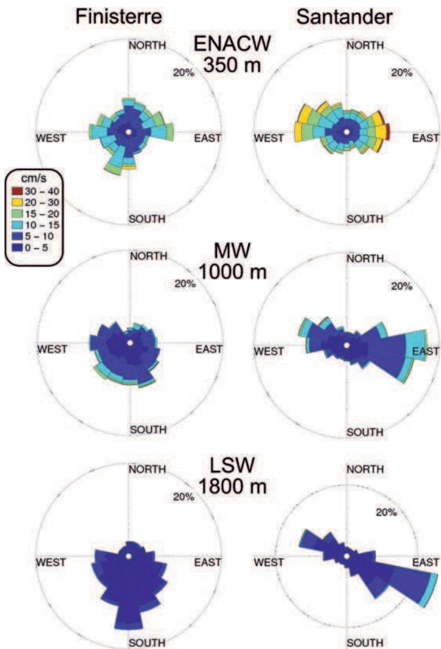
Figura 2.12. Patrones climatológicos de las corrientes profundas ( \text{cm s}^{-1} ) a los niveles de las Aguas Centrales (ENACW), Mediterránea (MW) y del Labrador (LSW) obtenidos a partir de los fondeos permanentes de VACLAN.
