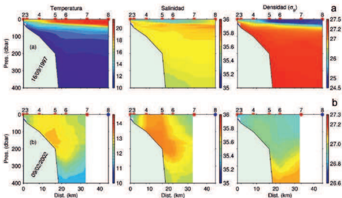
Figura 2.3. Registro de temperatura (°C), salinidad y densidad potencial en la sección hidrográfica de Santander bajo la influencia de un afloramiento intenso (a) y en una situación de IPC plenamente desarrollada (b).
