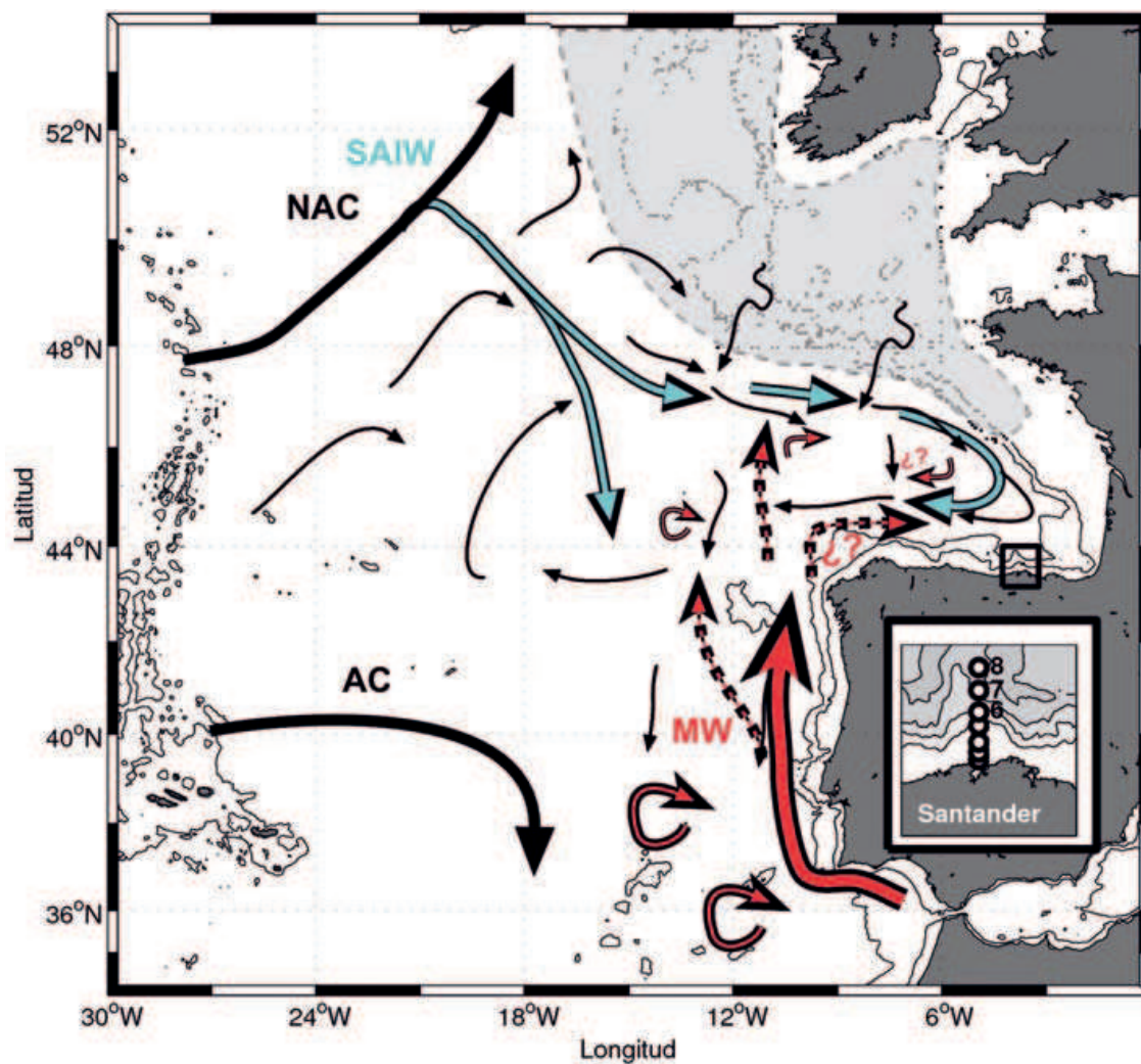
Figura 2.10. Composición a partir de diversas fuentes de los patrones principales de circulación de las Aguas Centrales (negro), hasta su base en el mínimo de salinidad (azul), y las Aguas Mediterráneas (MW, rojo) en el Golfo de Vizcaya y la parte adyacente del Atlántico norte. Se indican las corrientes Noratlántica y Azores (NAC y AC), el aporte de Aguas Subárticas Intermedias (SAIW), y las regiones de aporte por "cascading" (degradado en gris) en las plataformas continentales al norte del Golfo de Vizcaya. Los interrogantes indican incertidumbre sobre patrones generales al nivel de la MW en algunas zonas. Modificado de Gonzalez-Pola (2006).
