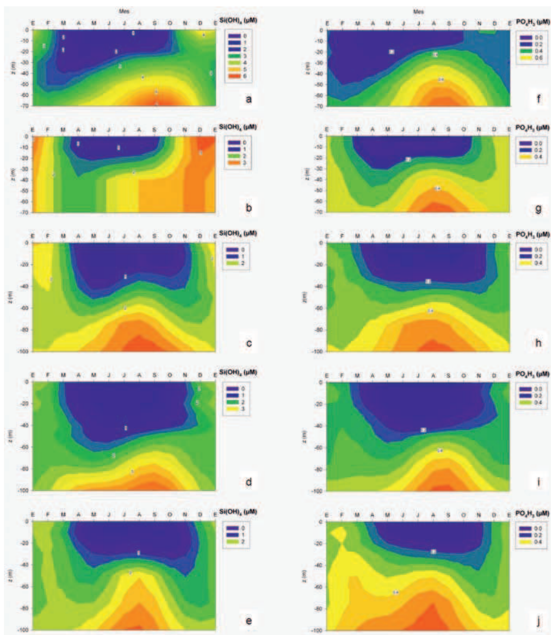
Figura 4.3. Ciclo estacional de concentraciones ( \mu\text{M} ) de silicato (izquierda, a-e) y de fosfato (derecha, f-j) en la estación intermedia de la plataforma en Vigo (a, f), A Coruña (b, g), Cudillero (c, h), Gijón (d, i) y Santander (e, j). La escala de variación en cada figura es diferente y ajustada al rango de datos.
