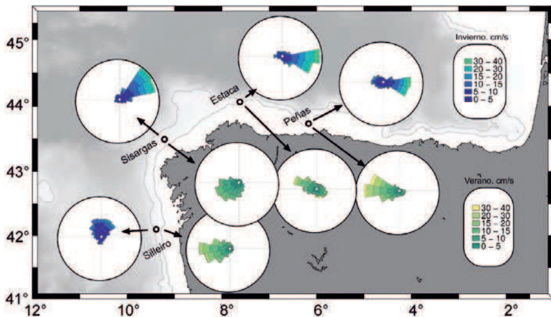
Figura 2.2. Rosas de corrientes superficiales en invierno y en verano a partir de la red de boyas DWN de Puertos del Estado localizadas en Galicia y en el mar Cantábrico. Valores en \text{cm s}^{-1} .
