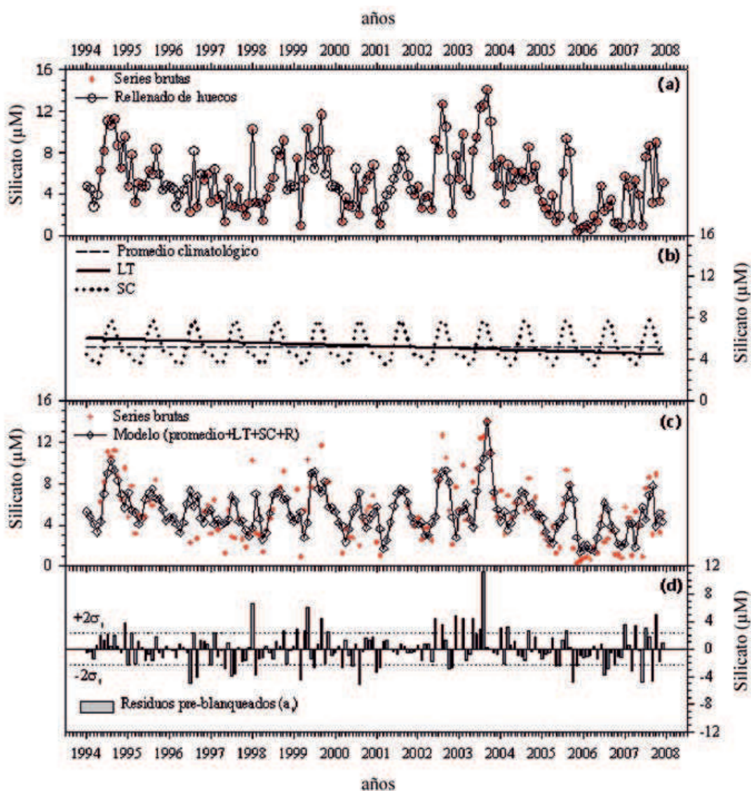
Figura I.1. Ejemplo de aplicación del modelo univariante de descomposición aditiva a la serie temporal de silicato a 35 m de profundidad en la estación 1 de la sección de Vigo. Se representan: serie bruta purgada y serie con huecos rellenados (a); componentes deterministas significativos ( p < 0.05 ) de las series: promedio climatológico, tendencia lineal (LT) y ciclo estacional (SC) como suma del primero y segundo armónicos del ciclo anual (b); serie bruta y modelo univariante de descomposición aditiva, donde R simboliza el componente autoregresivo descontado los residuos preblanqueados (c) y residuos preblanqueados del modelo, donde \sigma_t simboliza su desviación estándar (d).
