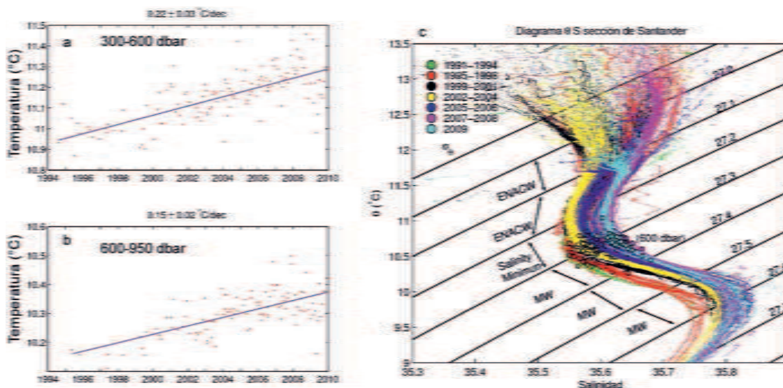
Figura 2.11. Evolución de la temperatura (°C) en la estación 7 de la sección de Santander en las capas representativas de las aguas centrales (a, 300-600 dbar, m) y de la parte superior del Agua Mediterránea (b, 600-950 dbar, m). Las líneas azules indican la tendencia lineal cuyo valor numérico ( \pm error estándar) figura en la parte superior. Se indica también la evolución del diagrama \theta S (c) distinguiendo diferentes periodos por medio de colores. Las líneas negras indican la densidad ( \sigma_\theta ).
