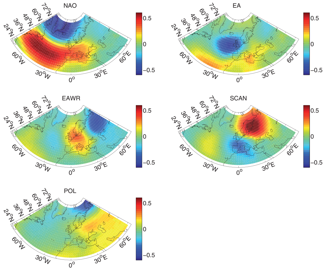
Figura 1.2. Patrones anuales de distribución espacial de los patrones de teleconexión atmosféricos (NAO, EA, EAWR, SCAN, POL). Se representa el valor del coeficiente de correlación entre el índice y la presión atmosférica a 500 hPa.
