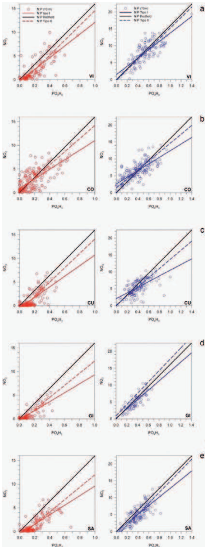
Figura 4.5. Relaciones estequiométricas entre el nitrato y el fosfato (N:P) en la superficie (10 m, rojo) y en la capa subsuperficial (70 m en VI y CO; 75 m en CU, GI y SA) para Vigo (a, VI), A Coruña (b, CO), Cudillero (c, CU), Gijón (d, GI) y Santander (e, SA). La línea negra indica las relaciones de Redfield (N:P = 16:1). Las líneas roja y azul indican el ajuste por regresión lineal a los datos (Tabla 4.6).
