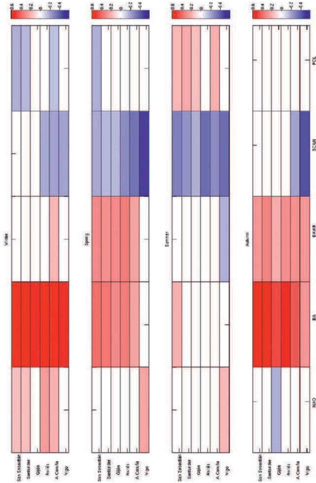
Figura 1.8. Correlaciones significativas entre la temperatura media mensual en las estaciones meteorológicas (AEMET) y los índices de teleconexión atmosférica.
