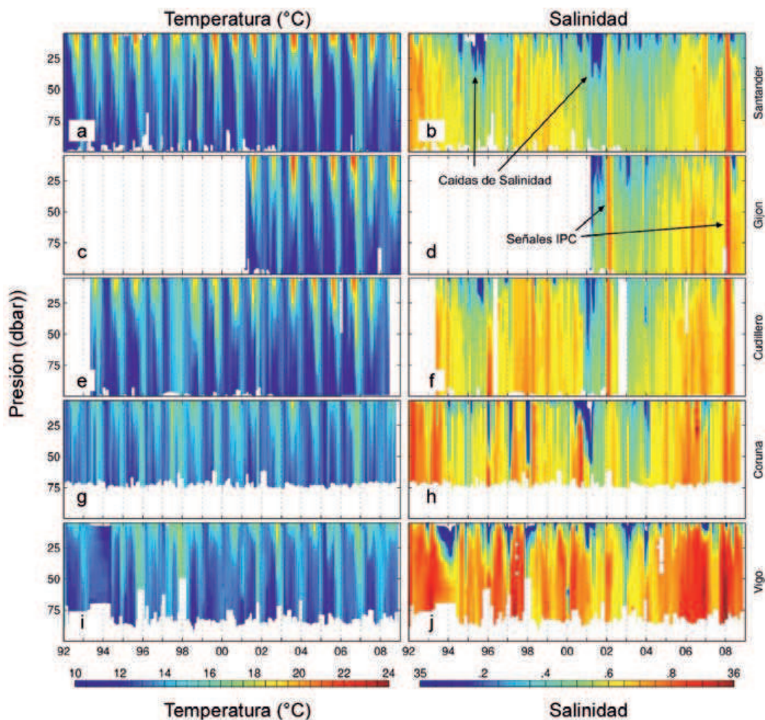
Figura 2.8. Variación temporal y vertical de temperatura (°C, a, c, e, g, i) y salinidad (b, d, f, h, j) en estaciones de plataforma media (~100 m) en las secciones de Vigo, A Coruña, Cudillero, Gijón y Santander. En Vigo y en Coruña las estaciones más profundas alcanzan tan sólo unos 75 m.
