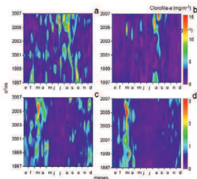
Figura 7.3. Distribución temporal de los valores medios semanales de la concentración de clorofila superficial ( \text{mg Cla m}^{-3} ) medida a partir de las observaciones del satélite SeaWifs en las distintas áreas seleccionadas: Rías de Vigo y Pontevedra (a), A Coruña (b), Asturias (c) y Santander (d). Nótese las distintas escalas para las zonas de Galicia (a, b) y del Mar Cantábrico (c, d). Modificado de Bode et al. (2011 b).
